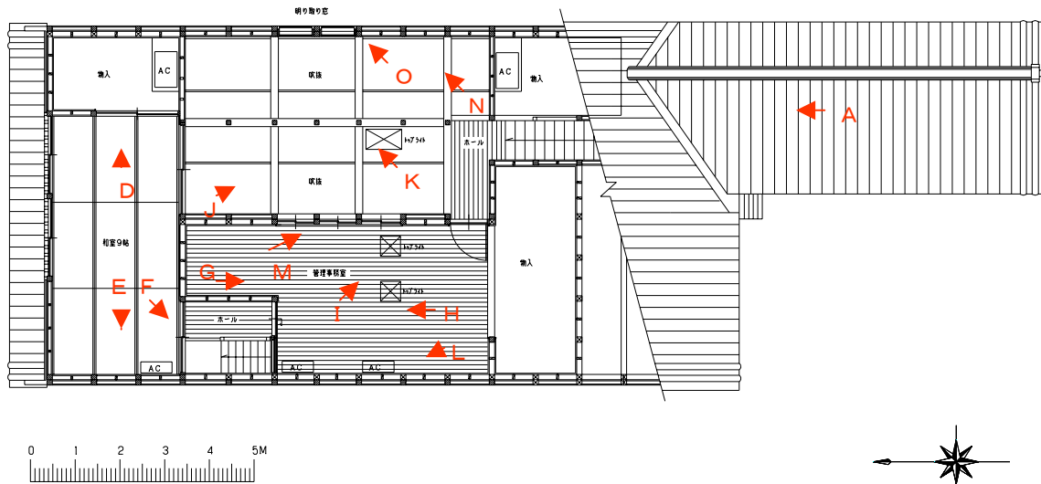
改修後 2階平面図
